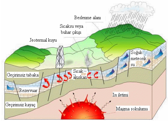
Şekil.1. Jeotermal sistemin şematik gösterimi
